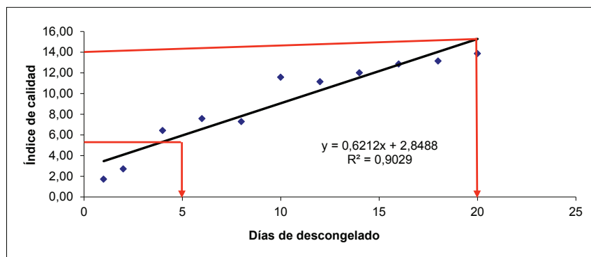
Figura 13. Curva de Calibración del Pez Sable HG (T) C/P
