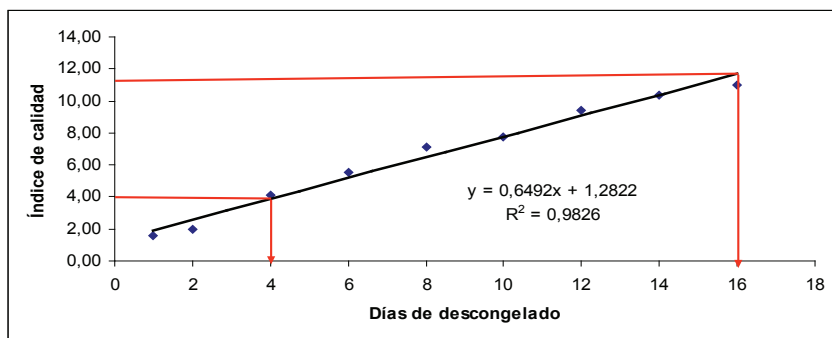
Figura 12. Curva de Calibración del Filete Talismán S/P
