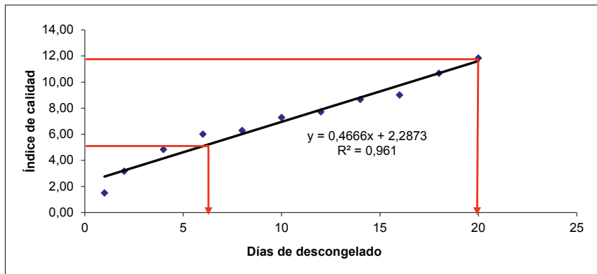
Figura 11. Curva de Calibración de la Platija Americana HG (T) C/P
