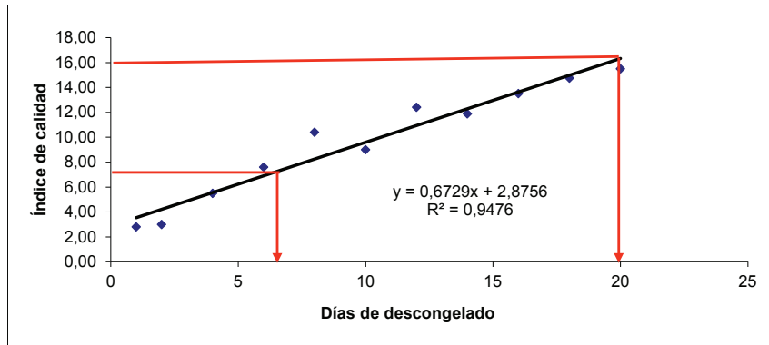
Figura 16. Curva de Calibración de la Rosada HG (T) C/P
