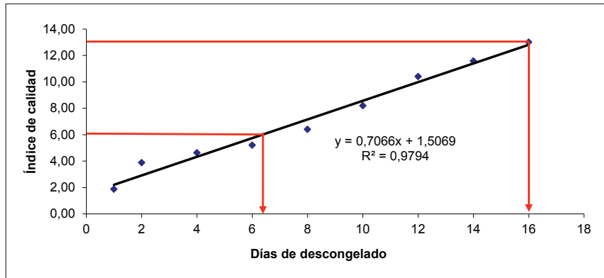
Figura 10. Curva de Calibración del Granadero HG (T) S/P
