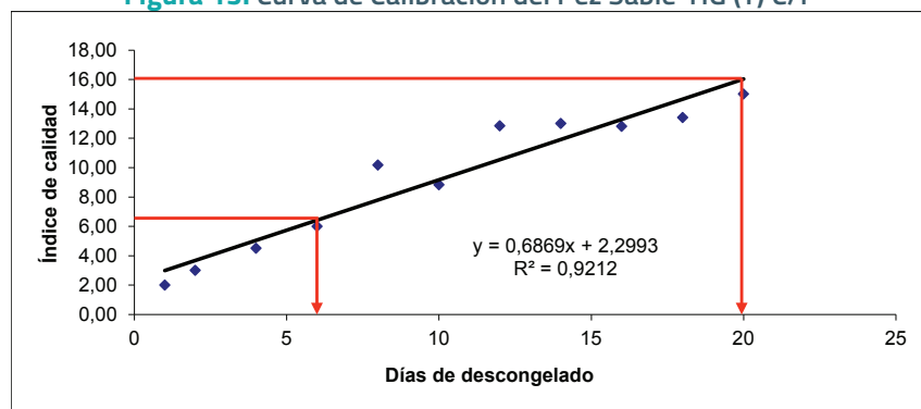
Figura 14. Curva de Calibración del Pez Palo HG (T) C/P
