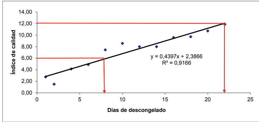
Figura 9. Curva de Calibración del Fletán Negro HG (T) C/P
